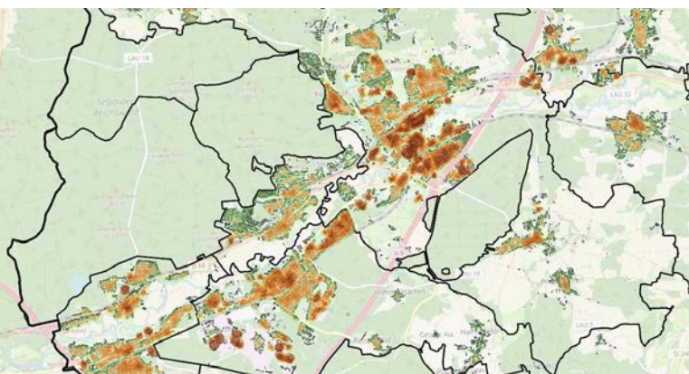
Auszug aus dem Digitalen Energienutzungsplan: Wärmedichtekarte auf Basis des gebäudescharfen Wärmekatasters (Bild: LK Nürnberger Land)
